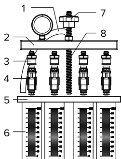
Diagrama de instalación del inyector de combustible de entrada superior
