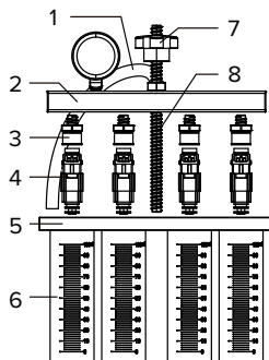
Installationsdiagramm für Kraftstoffinjektor oben einsetzen
