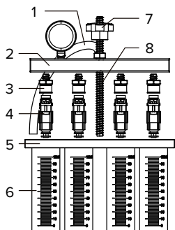
Diagramma di installazione dell'iniettore di carburante in alto
