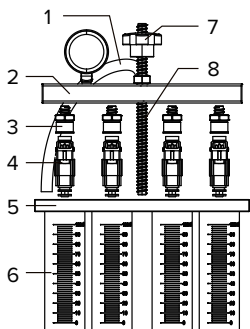
Diagramme d'installation de l'injecteur de carburant par le haut
